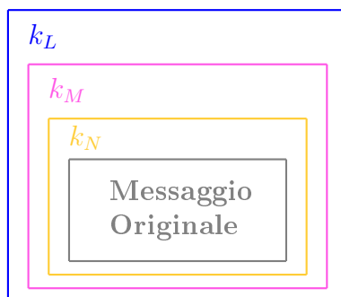
Figura 13: strati di cifratura TOR
